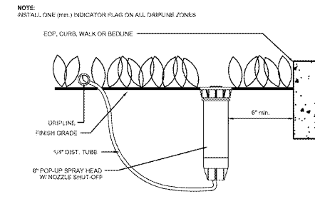
7 ZONE INDICATOR FLAG SCALE: NTS
