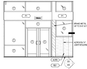
2 VESTIBULE ELEVATION A1.2 14" x 14"
