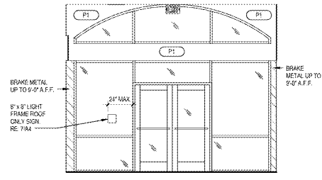
3 VESTIBULE ELEVATION A1.2 14" x 14"
