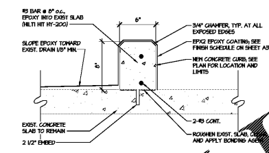
CURB DETAIL 5 SCALE: 1 1/2" = 1'-0"
